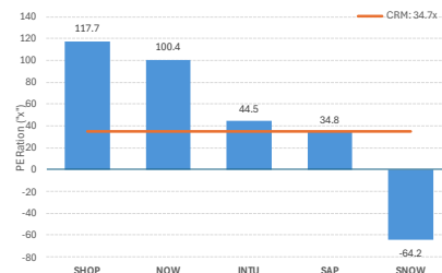
PE ratio
